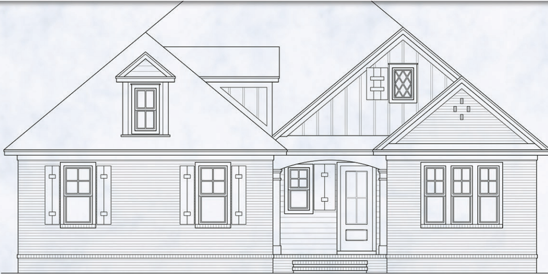
ELEVATION A
