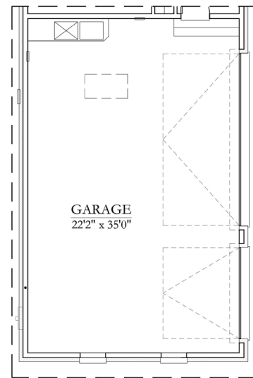
2 DOOR 3 CAR GARAGE ADD 274 SQ FT
