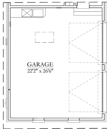
2 DOOR 2 CAR GARAGE ADD 77 SQ FT
