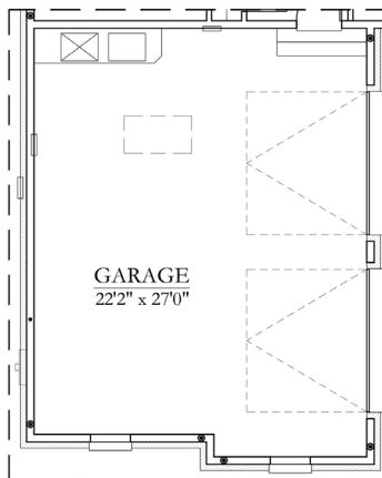
2 DOOR 2 CAR GARAGE ADD 77 SQ FT
